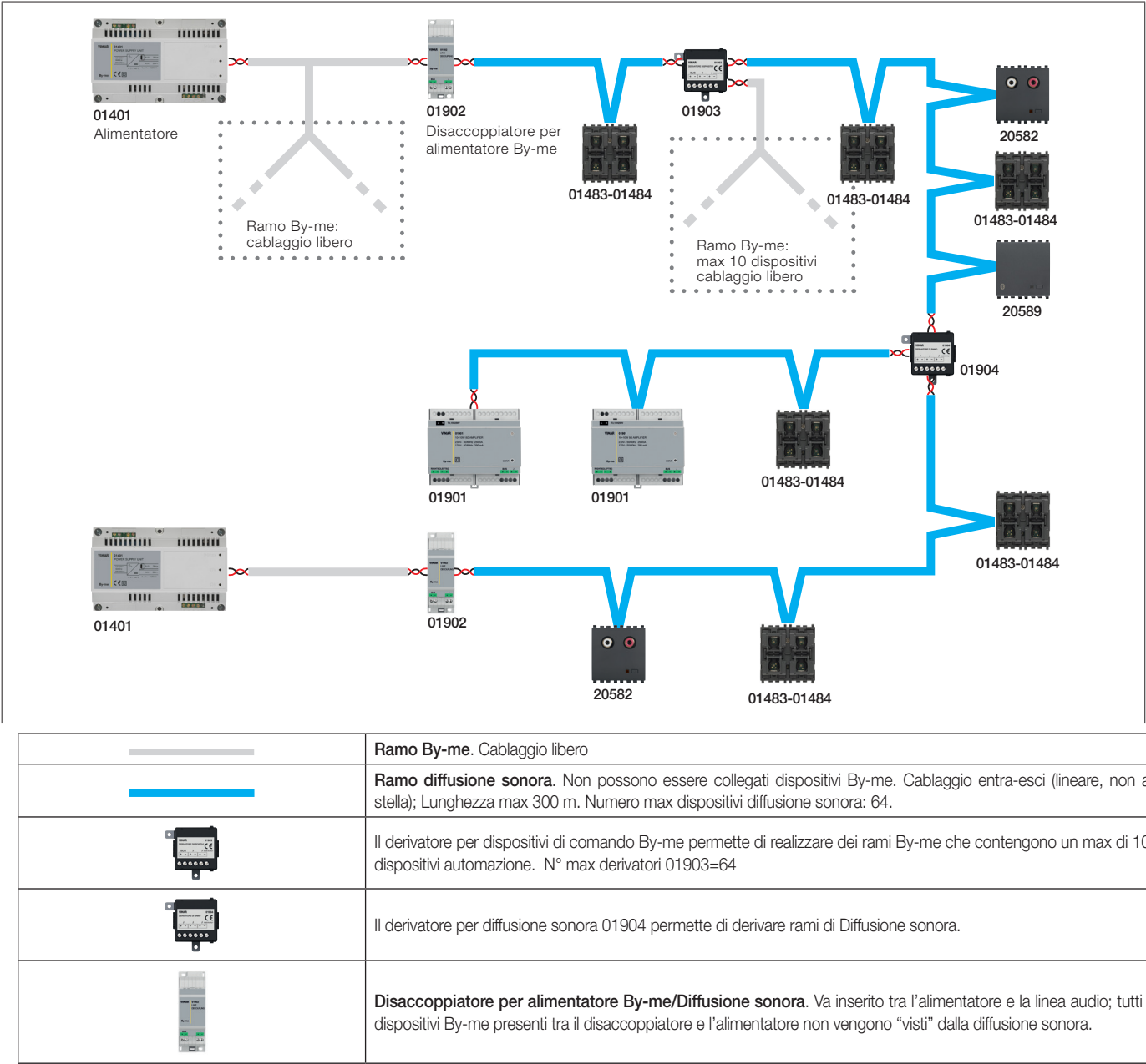
Esempio 3: diffusione sonora e automazione By-me sullo stesso ramo
