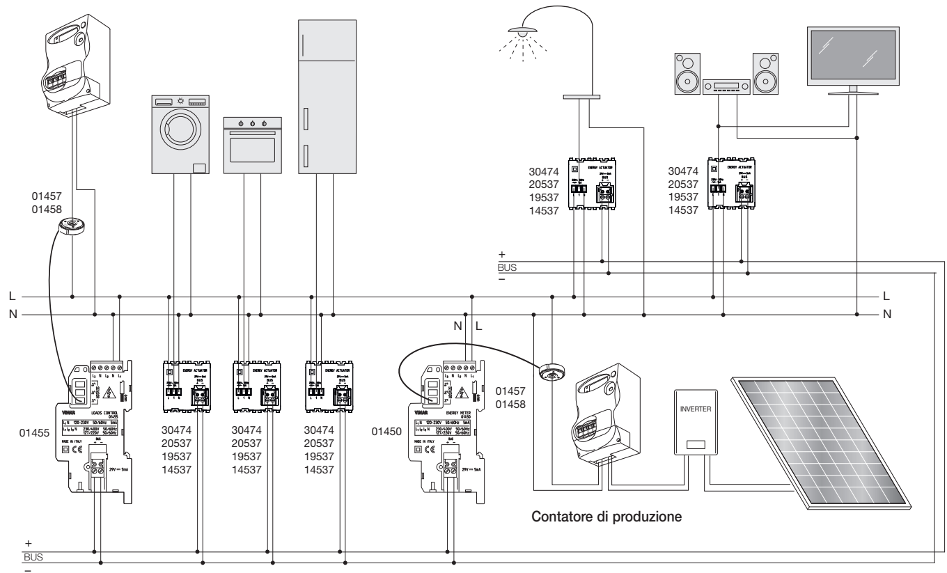
Contatore di scambio
